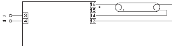
Wiring 1
