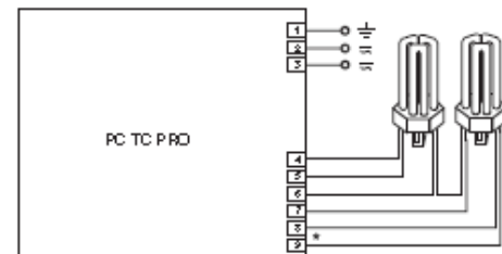
Wiring 12
