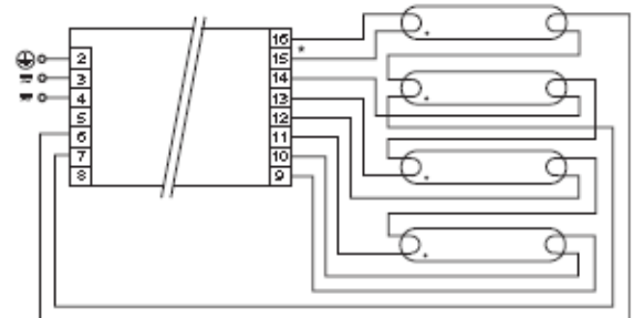
Wiring 12
