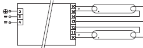
Wiring 7
