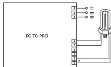
Wiring 11
