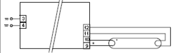
Wiring 4
