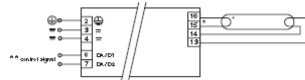
Wiring 13 & 14
