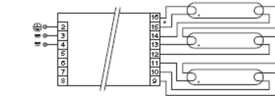
Wiring 9 & 10
