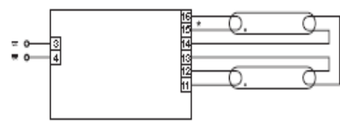
Wiring 3
