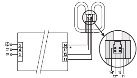
Wiring 8
