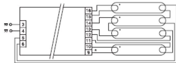
Wiring 6
