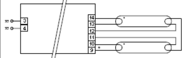
Wiring 6
