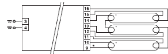
Wiring 5
